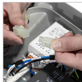
Konektory poke-yoke pro snadnou integraci do svítidel TECEO 1, které jsou odolné proti chybám.
